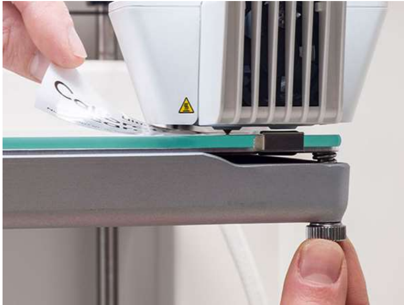
Réglage de la hauteur du plateau
